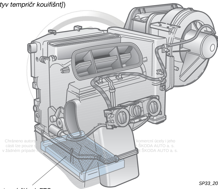
topný článek PTC doplňěk výměníku tepla topení ve vozidle
