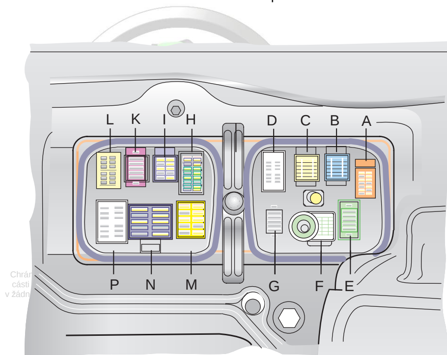
Kompaktní svorkovnice – pohled z motorového prostoru
